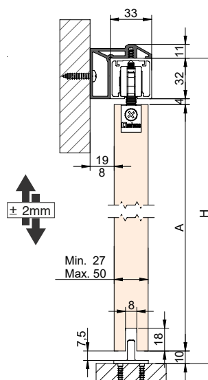
STAR + SEPARADOR | SEPARATOR | SÉPARATEUR A= H-47
