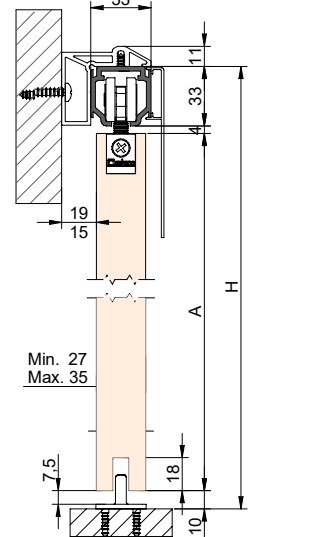
EXCELLENCE + SEPARADOR | SEPARATOR | SÉPARATEUR A= H-47
