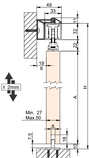
STAR + SEPARADOR | SEPARATOR | SÉPARATEUR A= H-65
