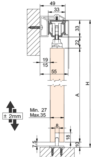
EXCELLENCE + SEPARADOR | SEPARATOR | SÉPARATEUR A= H-65
